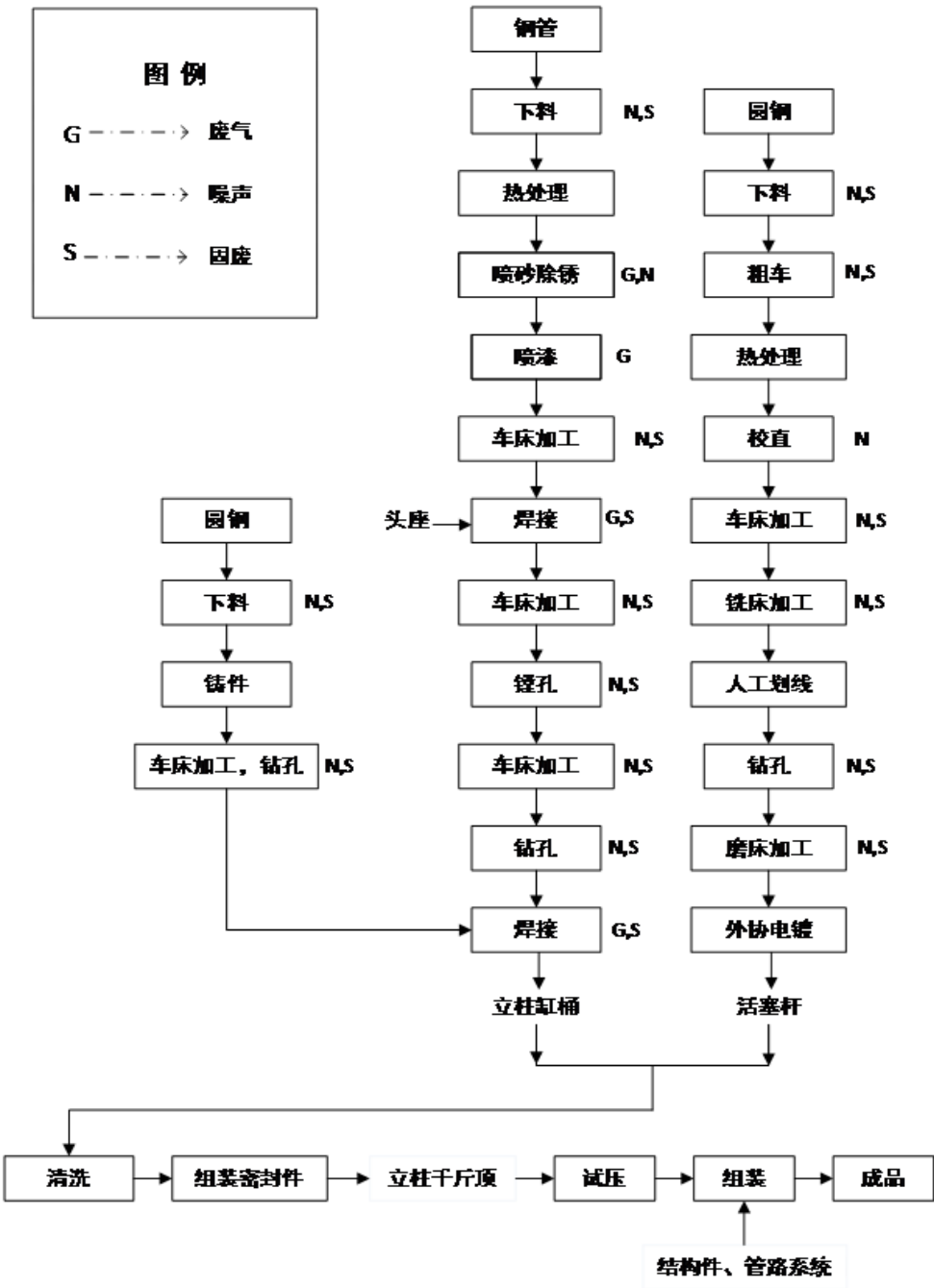
图 3-2 生产工艺流程图
