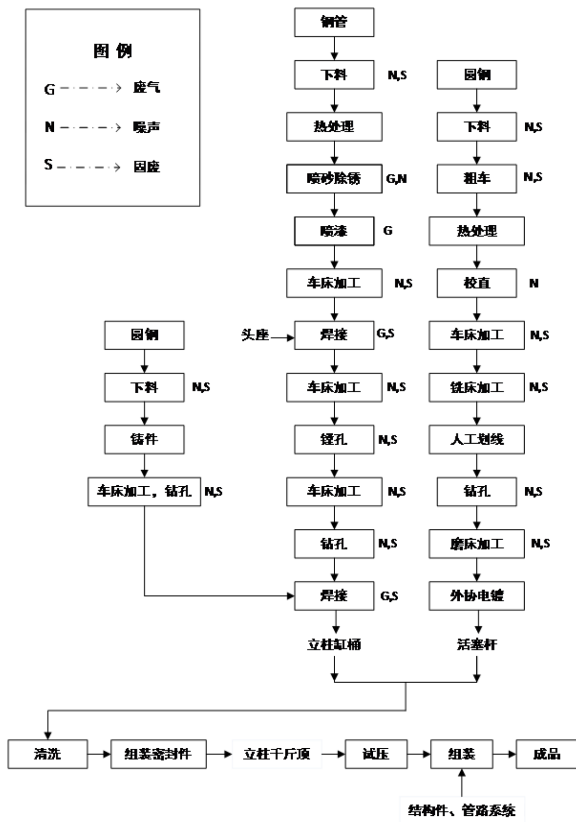
附件 4: 工艺流程图
